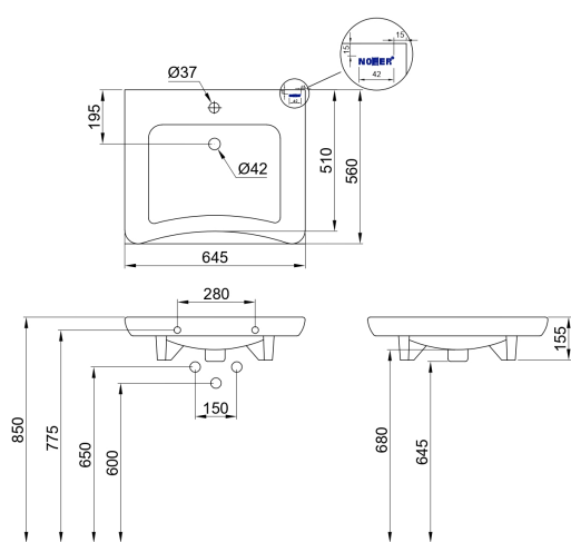
Esquema dimensional soporte
