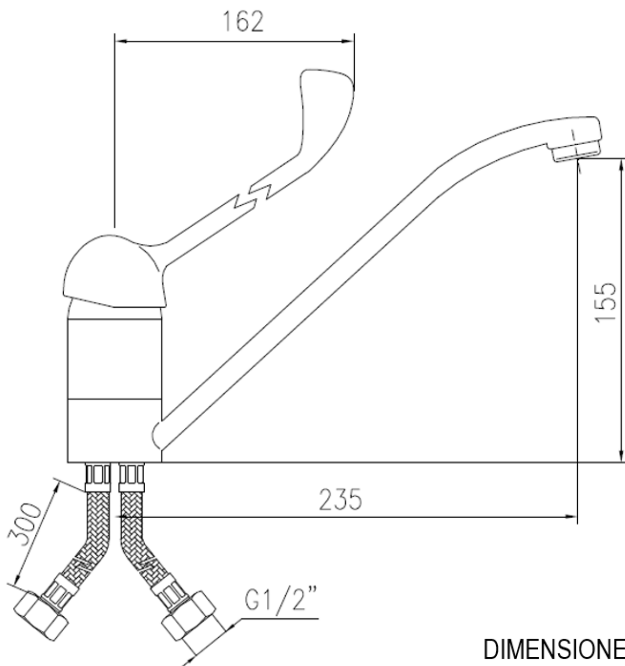
Esquema dimensional lavamanos
