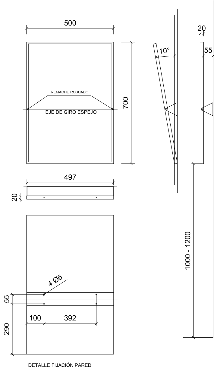
DETALLE FIJACIÓN PARED
